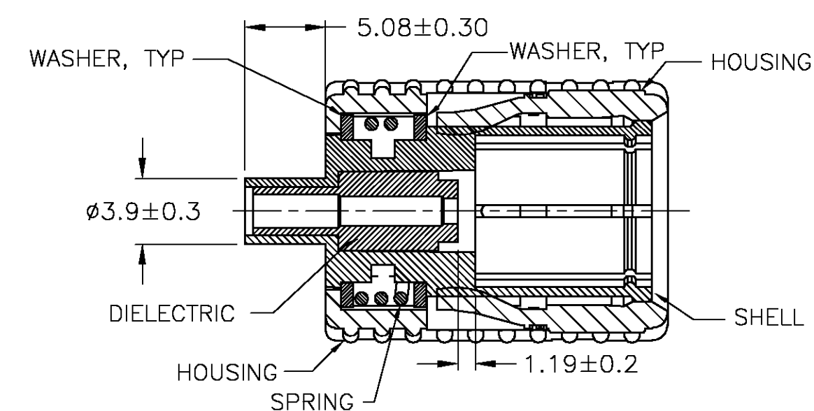
SECTION A-A 109763-3
