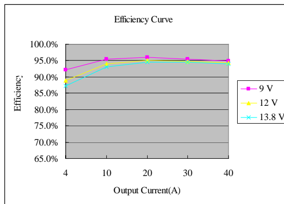
Vout = 5.0 V
