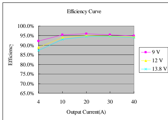
Vout = 5.0 V
