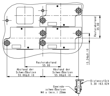
Einzelbefestigung
