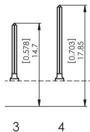
Wire-Wrap Termination □ 0.6 mm (0.024") Wire-Wrap Anschluss □ 0,6 mm
