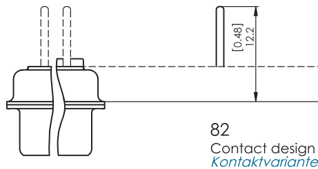
Straight PCB Termination Ø 1.0 mm (Ø 0.039") Gerader Leiterplattenanschluss Ø 1,0 mm
