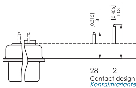
Straight PCB Termination Ø 0.76 mm (Ø 0.030") Gerader Leiterplattenanschluss Ø 0,76 mm
