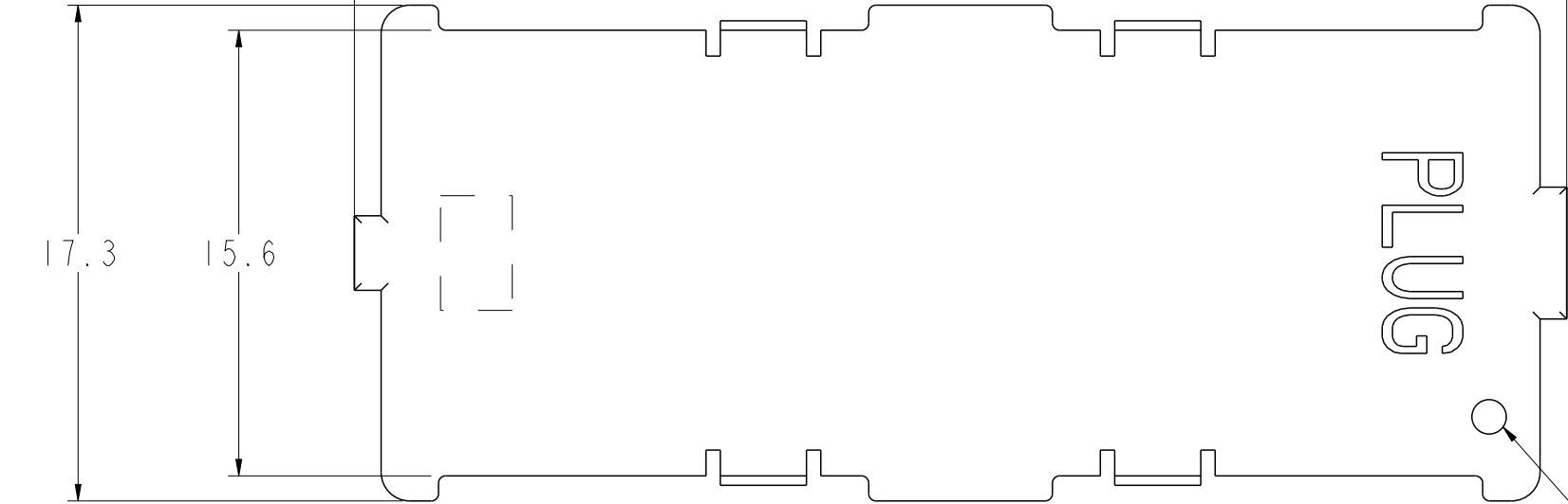
SCALE 4:1
