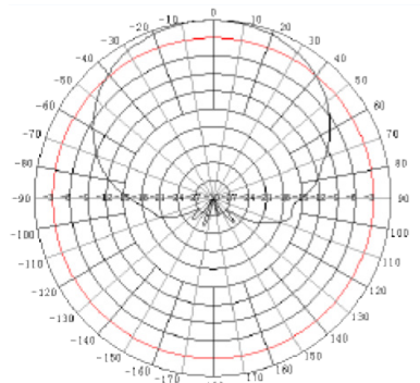
1800 MHz H-Plane
