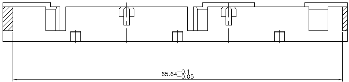
SECTION A-A
