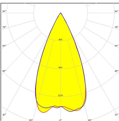
CP16109_CARMEN-50-W-C
