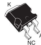
D²PAK STPSC606G
