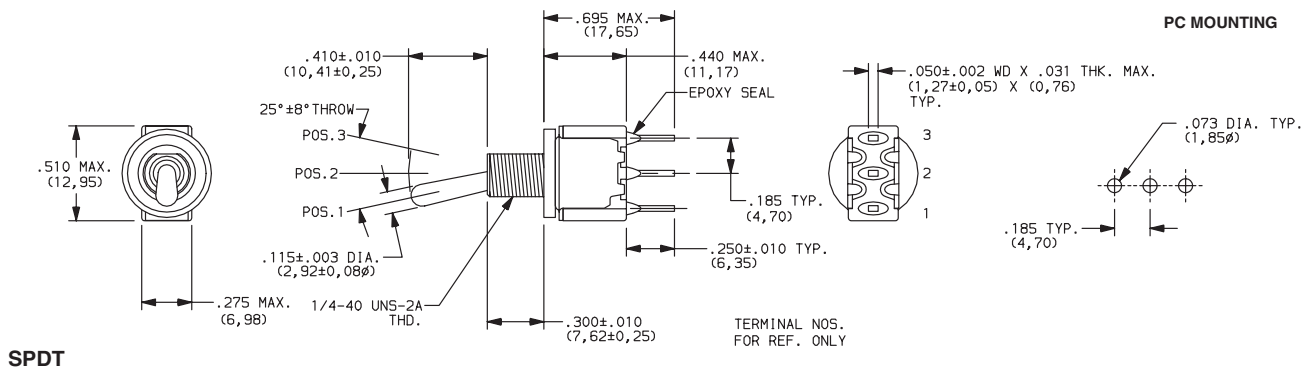
SPDT
