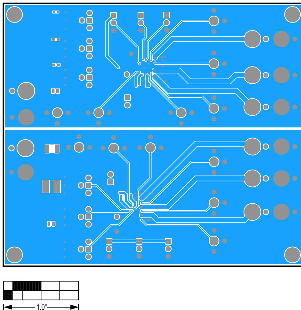
MAX17270 EV PCB—Bottom Layer
