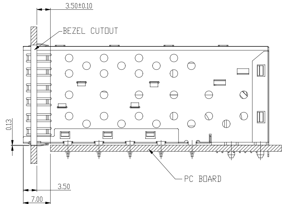
SECTION A-A
