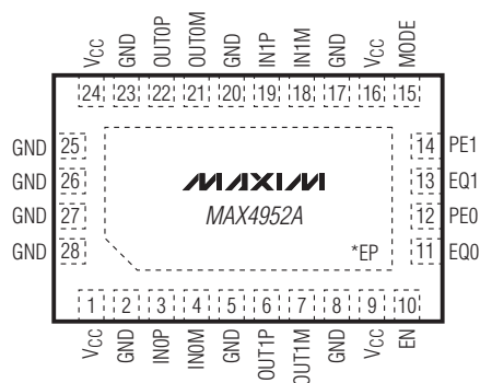
TQFN
