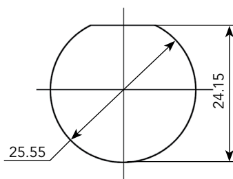
Jam Nut Receptacle - UTS7
