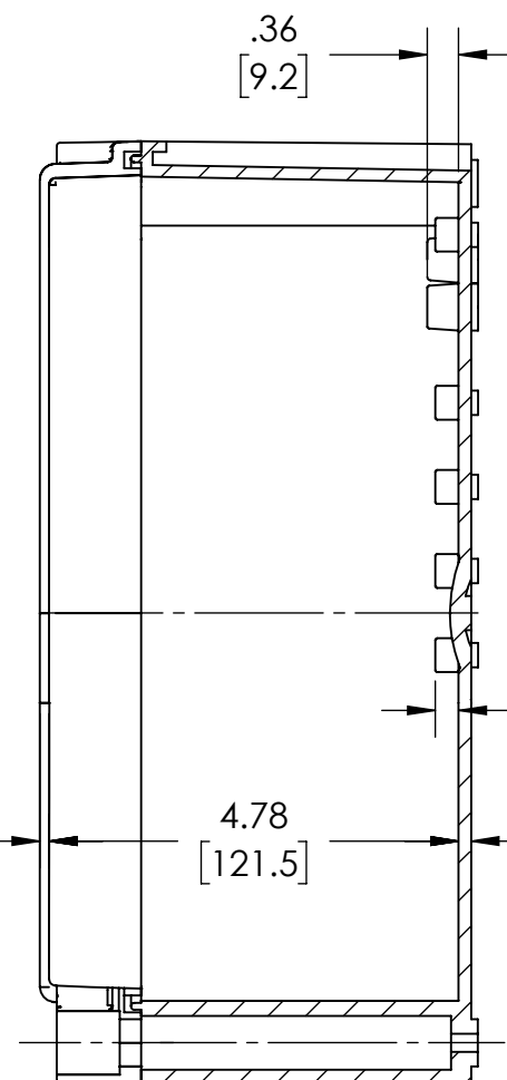
SECTION A-A
