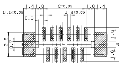
基板取付寸法 (奇数ピン)
