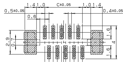
基板取付寸法（偶数ピン）
