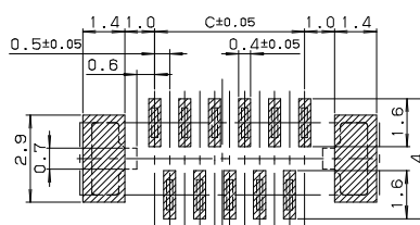
基板取付寸法（奇数ピン）
