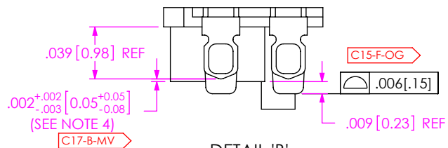
DETAIL 'B' SCALE 10 : 1
