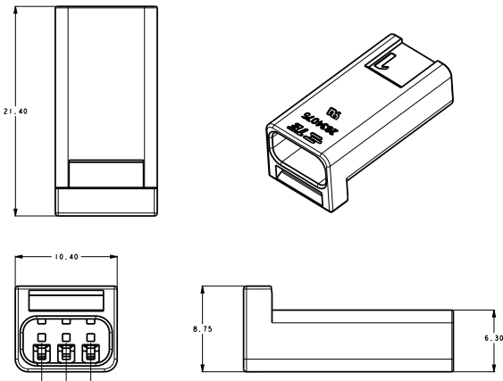
Receptacle
