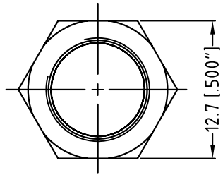
METAL NUT
