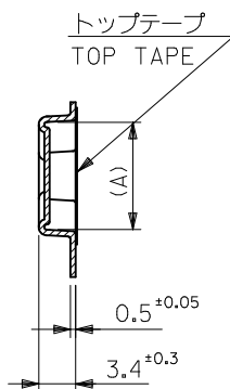
SECT.V-V
