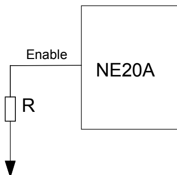
Fig. 18. Enable POR circuit.
