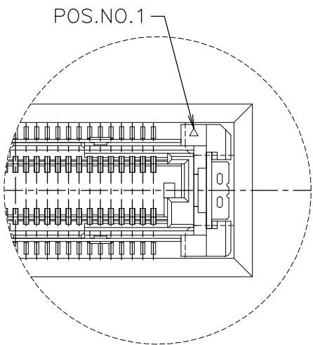
DETAIL E (SCALE 4:1)
