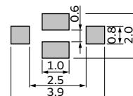
NFM3DCC/3DPC
