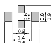
NFM21CC/21PC
