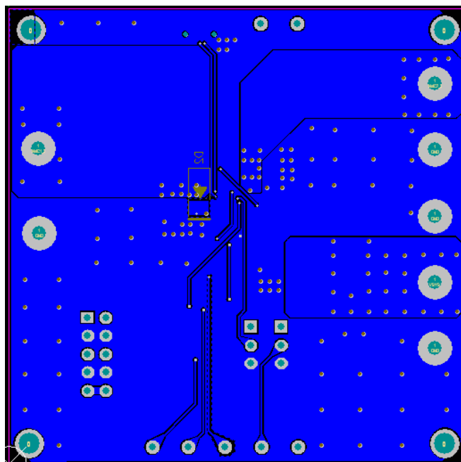
Figure 2—Bottom Layer
