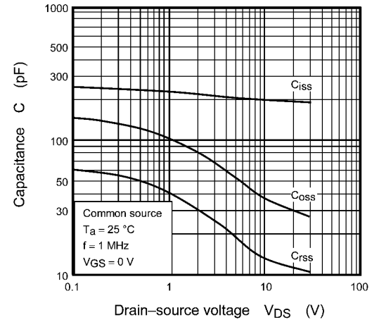
Fig. 7.10 C - V DS
