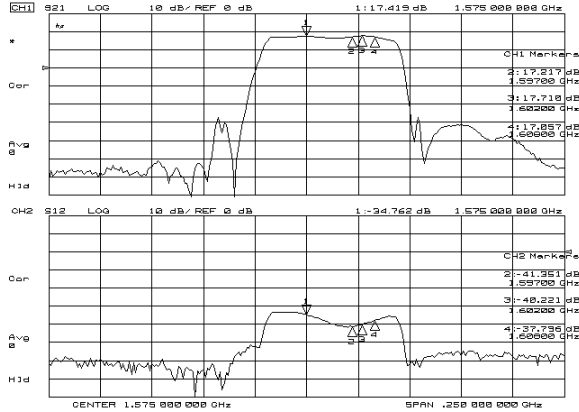
S21, S12
