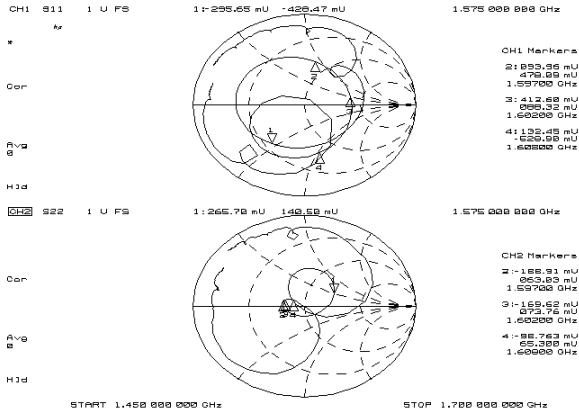
Zin, Zout
