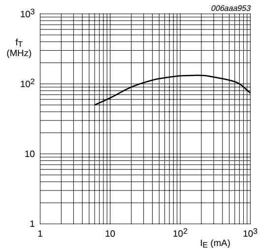
T_{amb} = 25\text{ }^{\circ}\text{C} ; V_{CE} = -2\text{ V}
