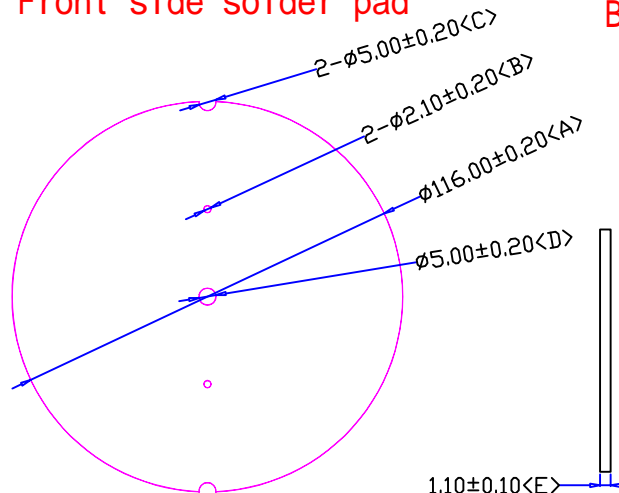
外形圖 Dimension
