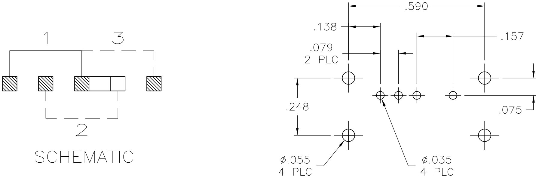
P.C.B. LAYOUT
