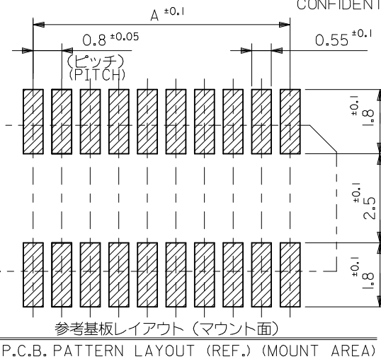
注記 NOTES 1. 嵌合相手 : 52465.52588 シリーズ MATES WITH : 52465.52588 SERIES 2. △エッジの 1/2 へ隣接するピンに ♯ の位置を示す。 SHOW POSITION FROM ♯ OF WAFER TO ♯ OF ADJACENT PINS. 3. ELV 及び RoHS 適合品。 ELV AND ROHS COMPLIANT. 4. テール平坦度 : 0.1MAX. COPLANARITY : 0.1MAXIMUM
