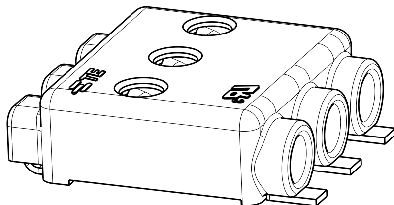
2213301-3 SCALE 6:1
